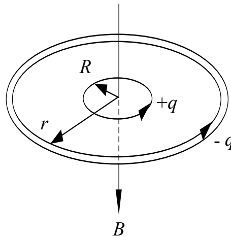
Рис. 2. Экваториальное сечение модели шаровой молнии, выделяющее кольца на токовых оболочках с фероидальной формой. R – радиус вращения ионов в равновесной оболочке вокруг магнитного поля с индукцией B , r – радиус внешней электронной оболочки.
